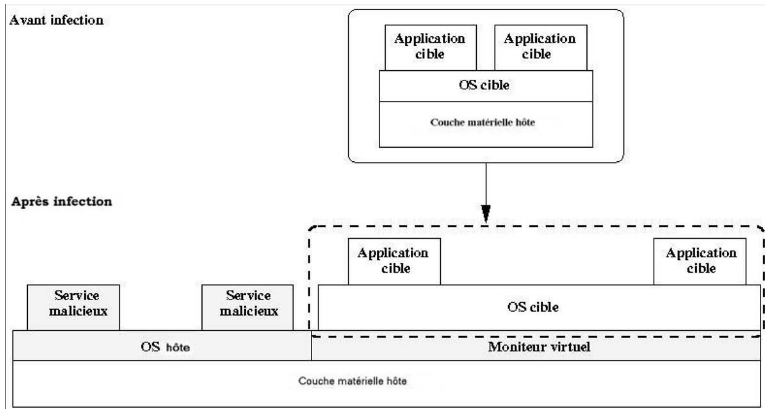
Figure 7.3 – Principe général du rootkit SubVirt [75].
