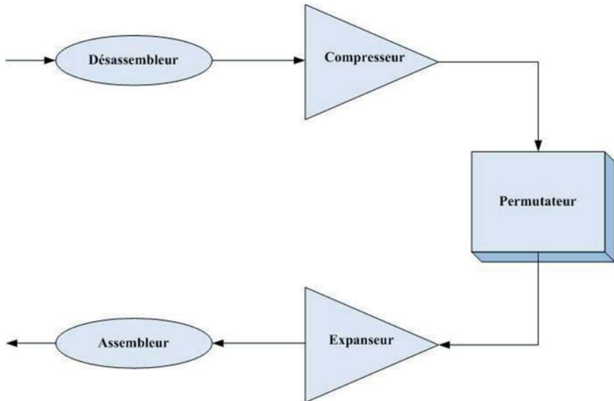
Figure 6.3 – Structure générale d'un moteur métamorphe
