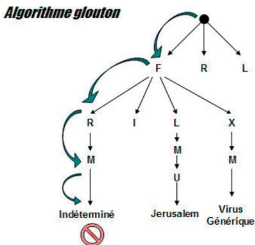
Figure 3.3 – Détection du virus Jérusalem par algorithme glouton (TbScan)
