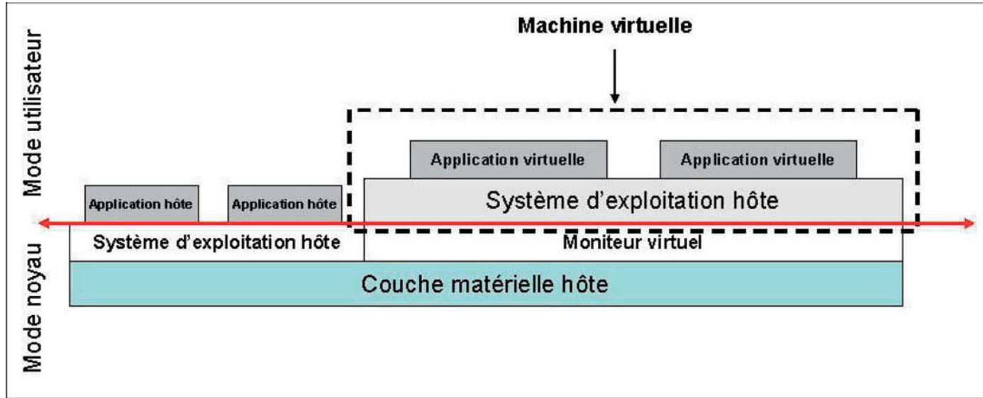
Figure 7.2 – Structure d'un moniteur virtuel (type VMware ou VirtualPC) [75].
