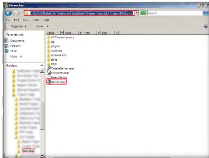
FIGURE 10.10: click server.exe
